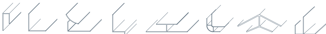
Moldura en J Ángulo exterior Bovedilla interior Moldura de base Divisor en H Ángulo interior/exterior 45 Divisor en H Moldura en F
